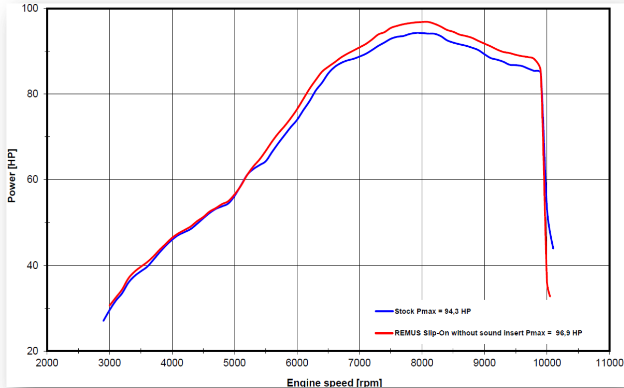
Leistungsdiagramm / Dyno chart – Slip on- Racing
